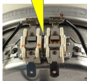
Thermostat de sécurité
